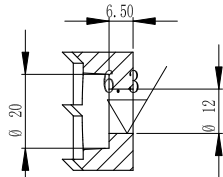
剖面 A-A
