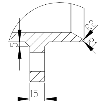
局部视图 B 比例 1 : 2
