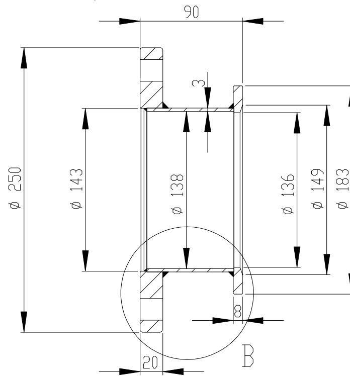
剖面 比例 1 : 3
