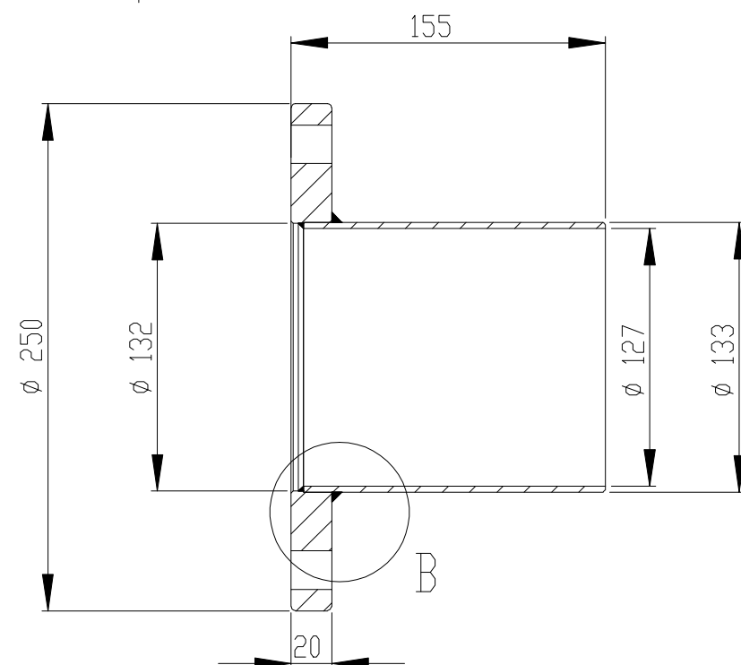
剖面 比例 1 : 3
