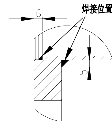
局部视图 B 比例 2 : 3
