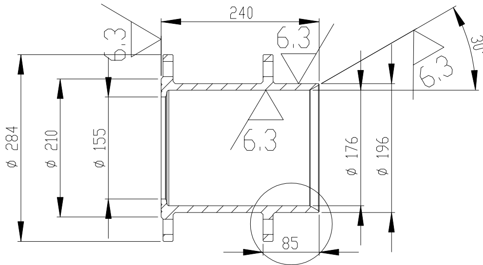
剖面 A-A
