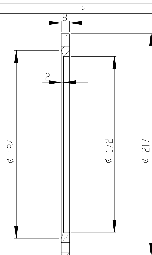
剖面 A—A
