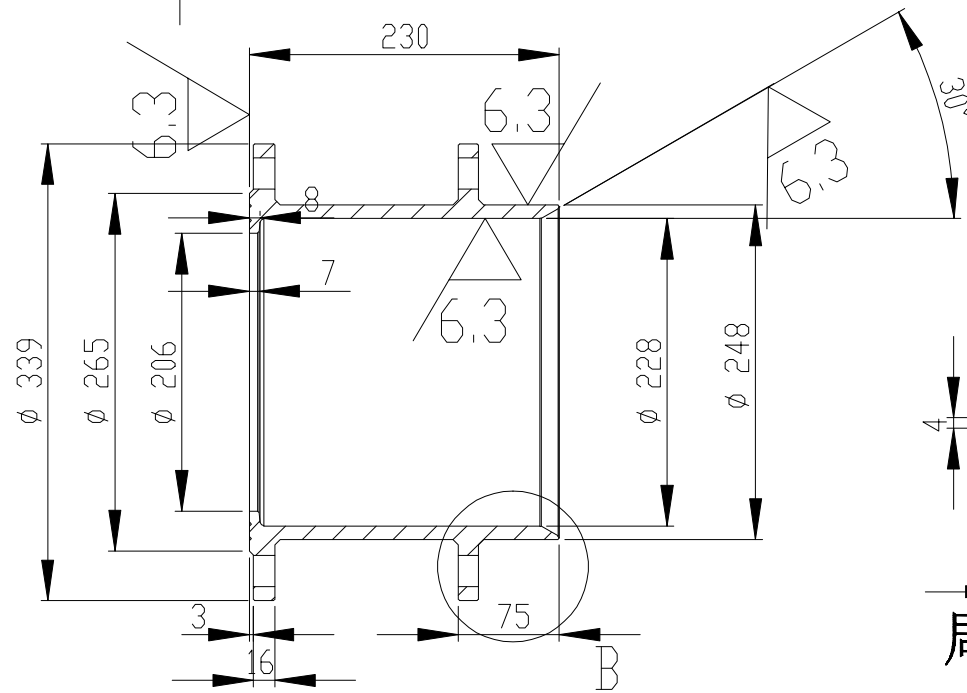
剖面 A-A
