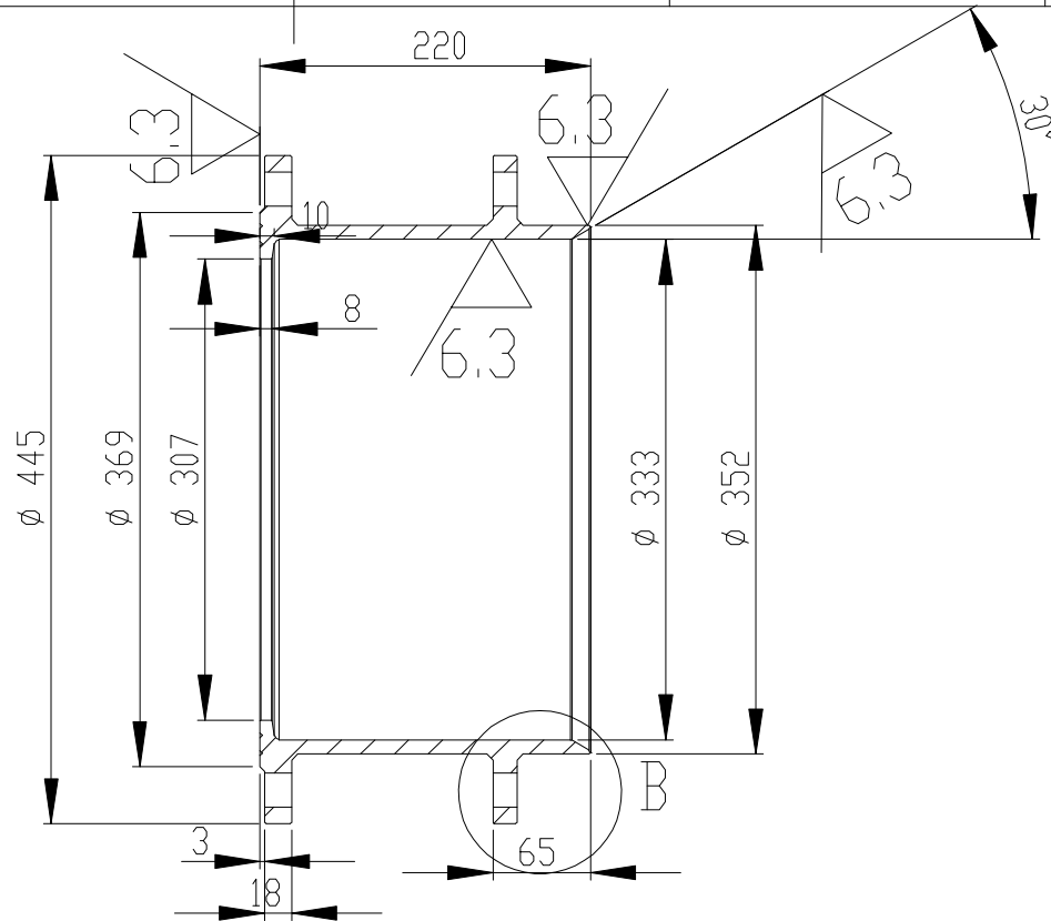
剖面 A-A
