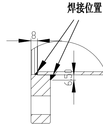
局部视图 B 比例 2 : 5
