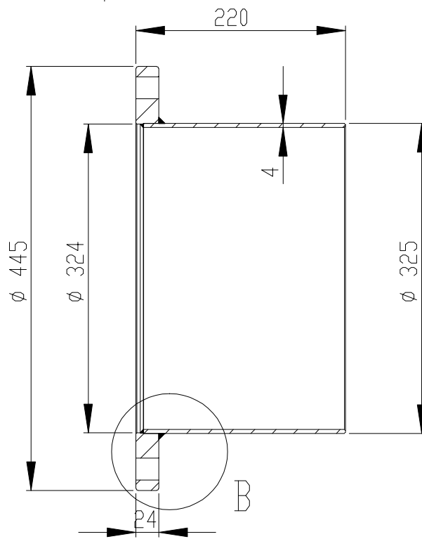
剖面 A-A
