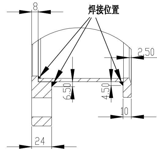
局部视图 B 比例 2 : 5
