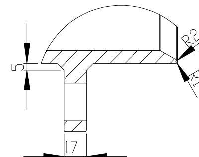
局部视图 B 比例 2 : 5
