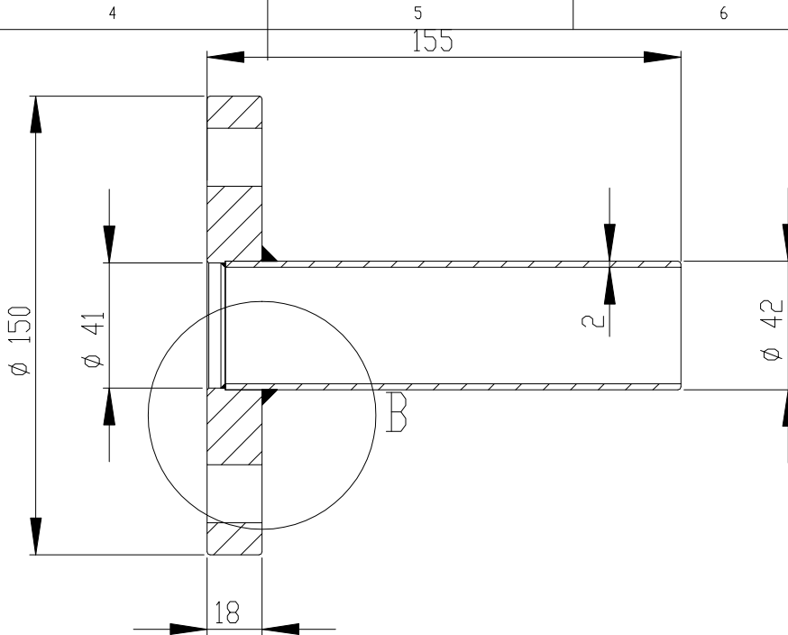
剖面 A-A
