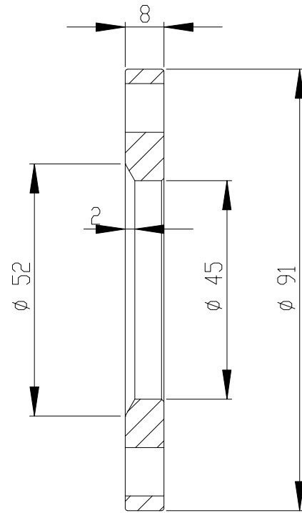
剖面 A-A
