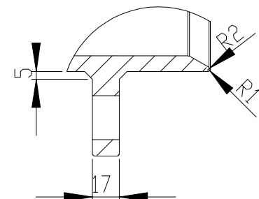
局部视图 B 比例 1 : 3
