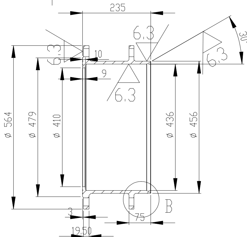
剖面 A-A 比例 1 : 7
