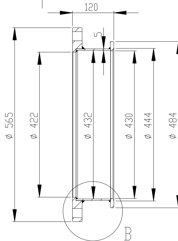
剖面 比例 1 : 6
