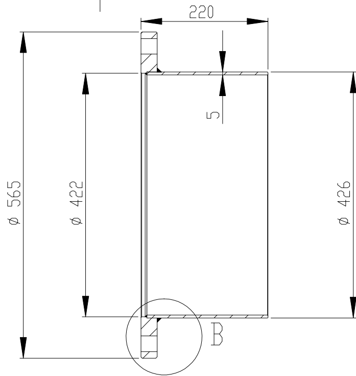
剖面 A-A 比例 1:6
