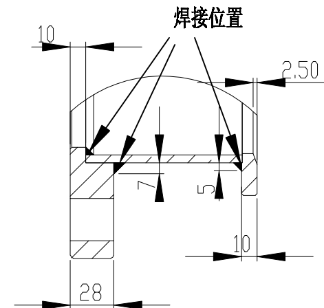
局部视图 B 比例 1 : 3
