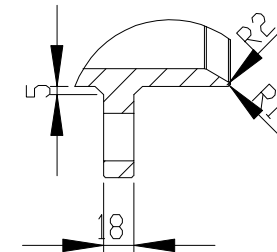
局部视图 B 比例 1 : 4
