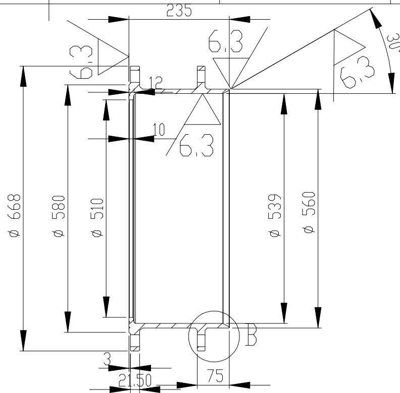
剖面 A-A 比例 1 : 8
