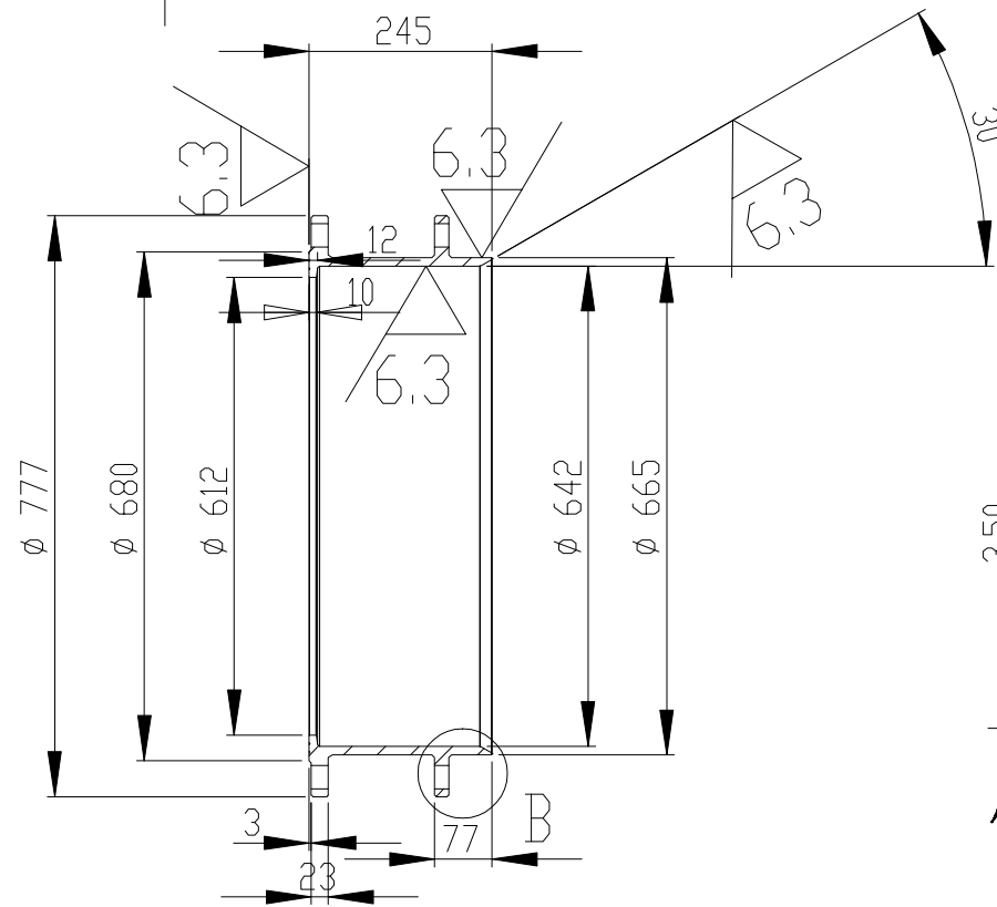
剖面 A-A
