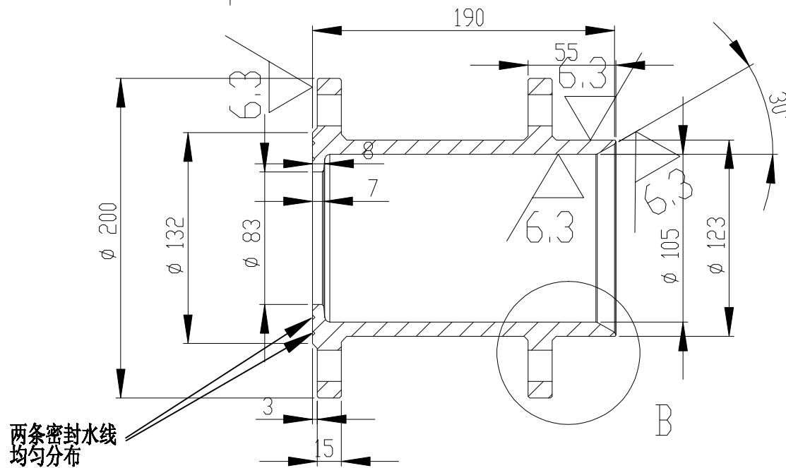
剖面 A-A 比例 1 : 3
