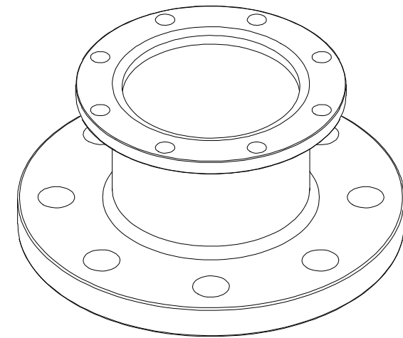
局部视图 B 比例 2 : 2.5
